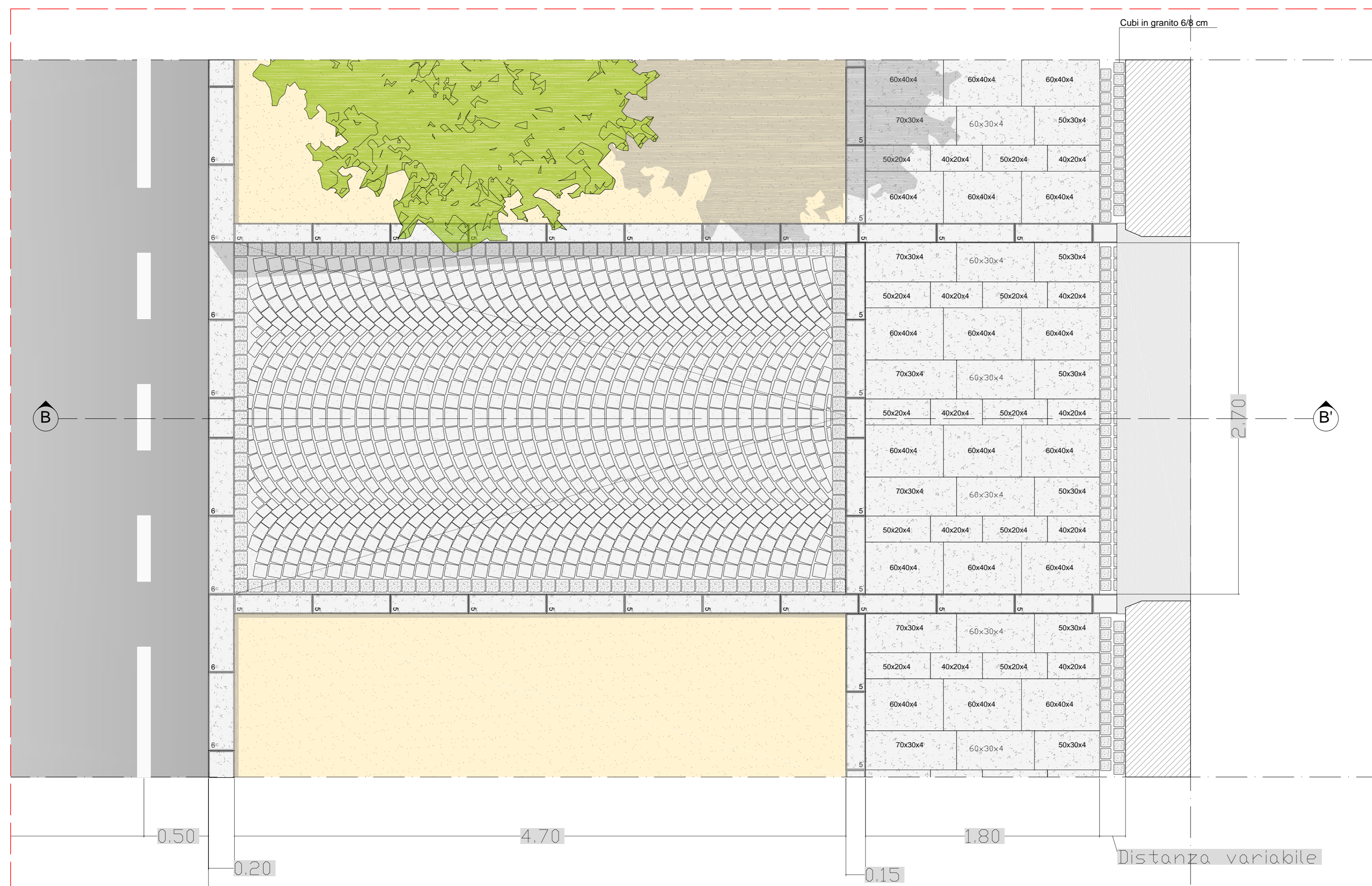
Pianta di posa della pavimentazione dei passi carrabili in cubi di in granito chiaro 10x10 cm (lato destro dir. viale S. Avendrace) - scala 1:100
