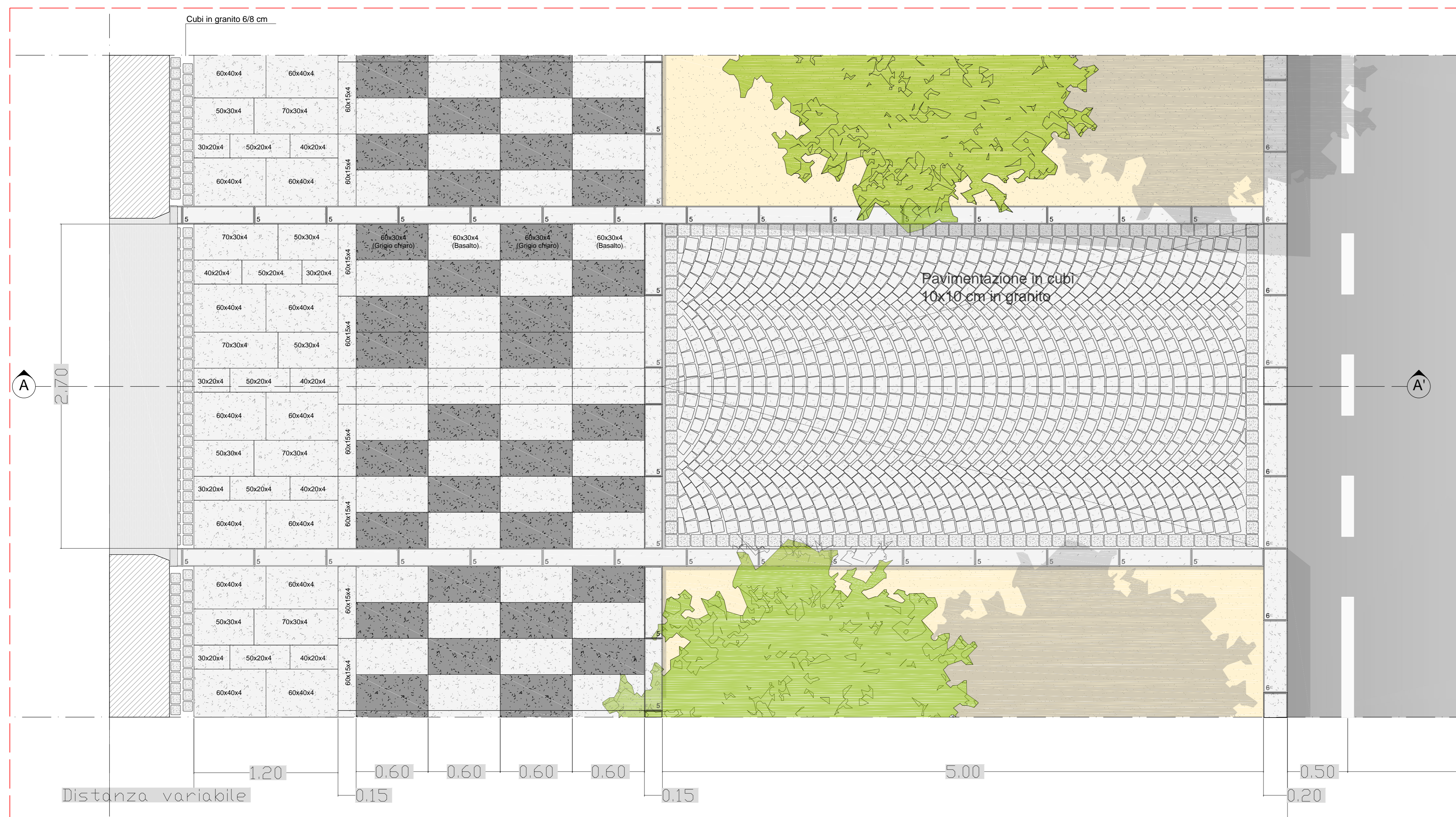
Pianta di posa della pavimentazione dei passi carrabili in cubi di in granito chiaro 10x10 cm (lato sinistro dir. viale S. Avendrace) - scala 1:100
