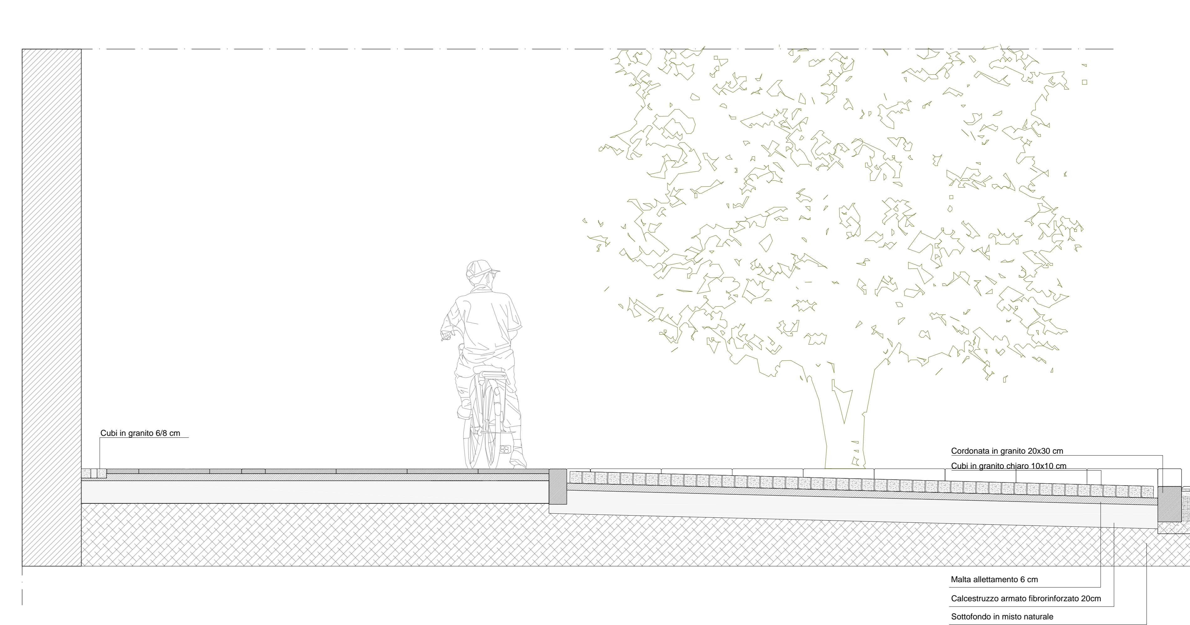
Sezione B-B' - scala 1:100
