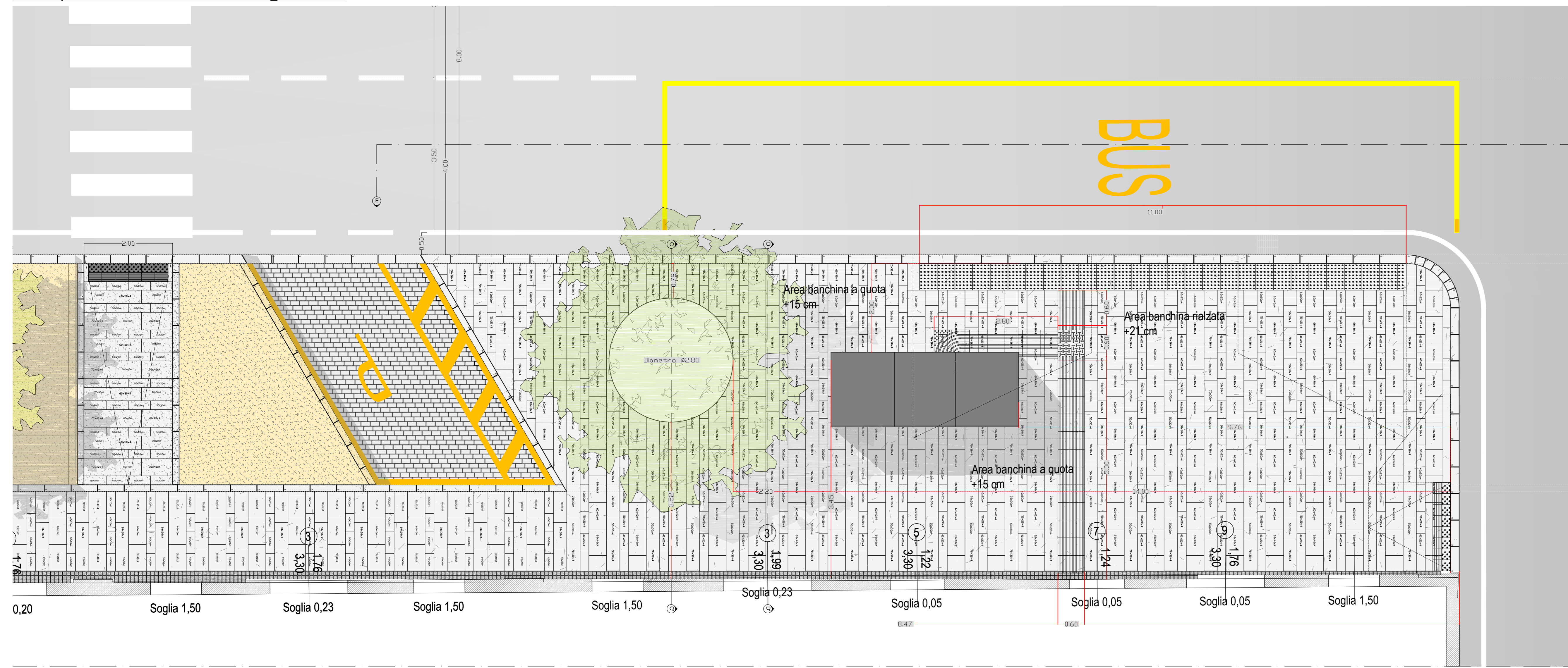
Stralcio planimetrico banchina di attesa TPL_scala 1:200
