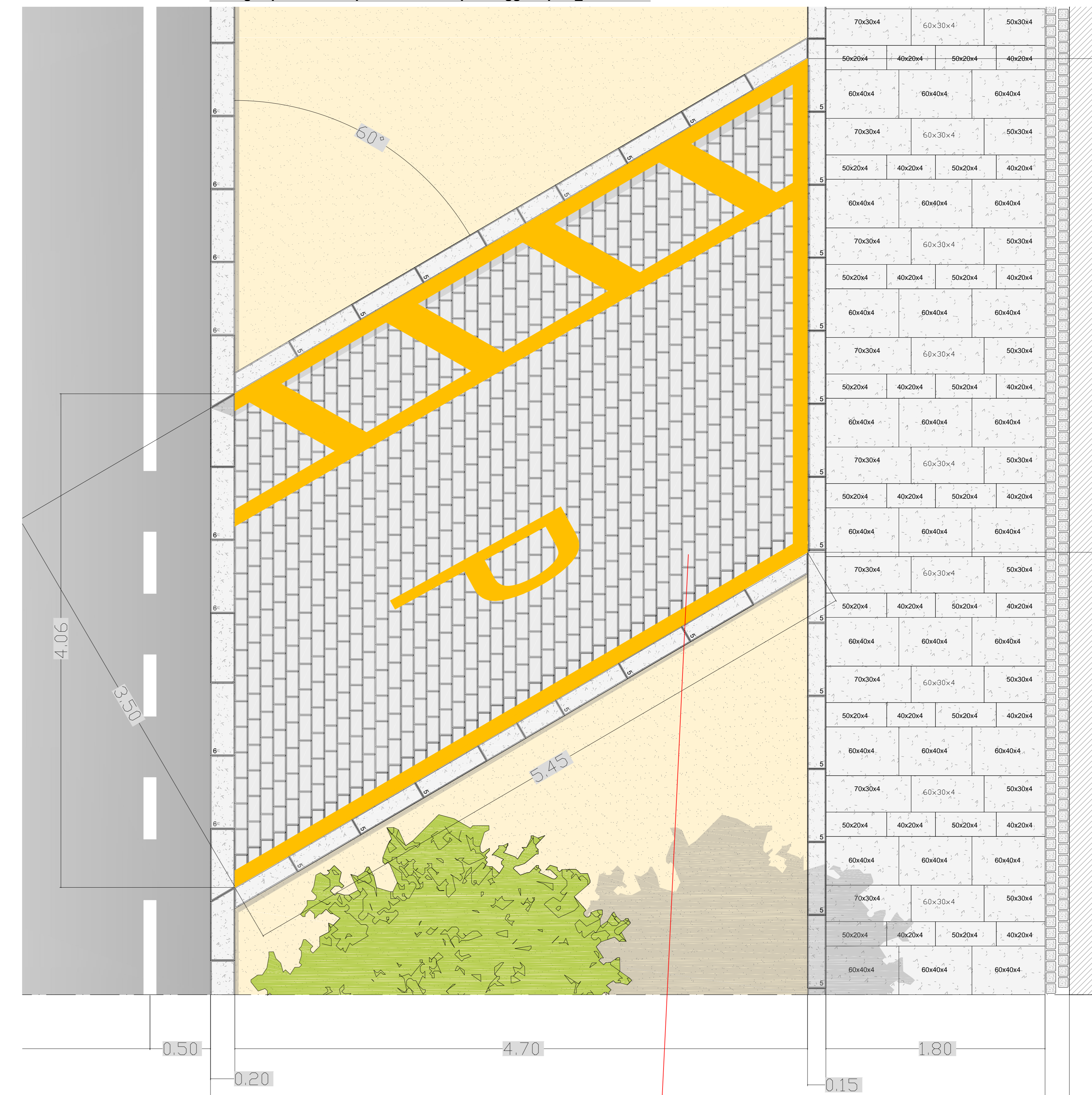
Dettaglio planimetrico pavimentazione parcheggi a spina_scala 1:50
