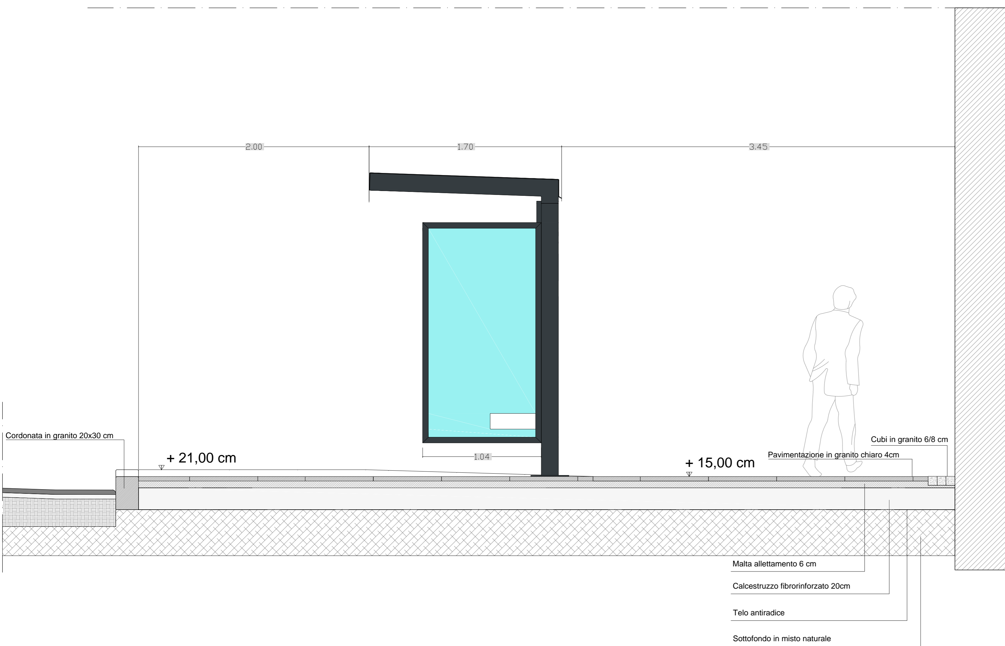
Sezione C-C'_scala 1:100
