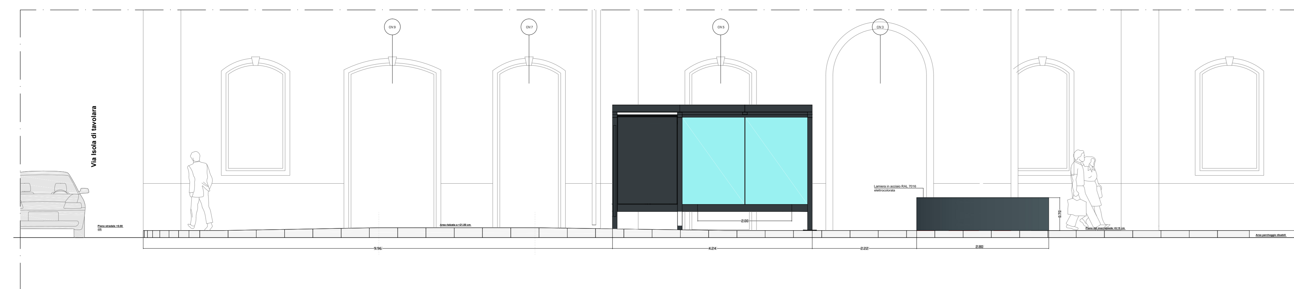
Prospetto E-E' banchina di attesa TPL_scala 1:200
