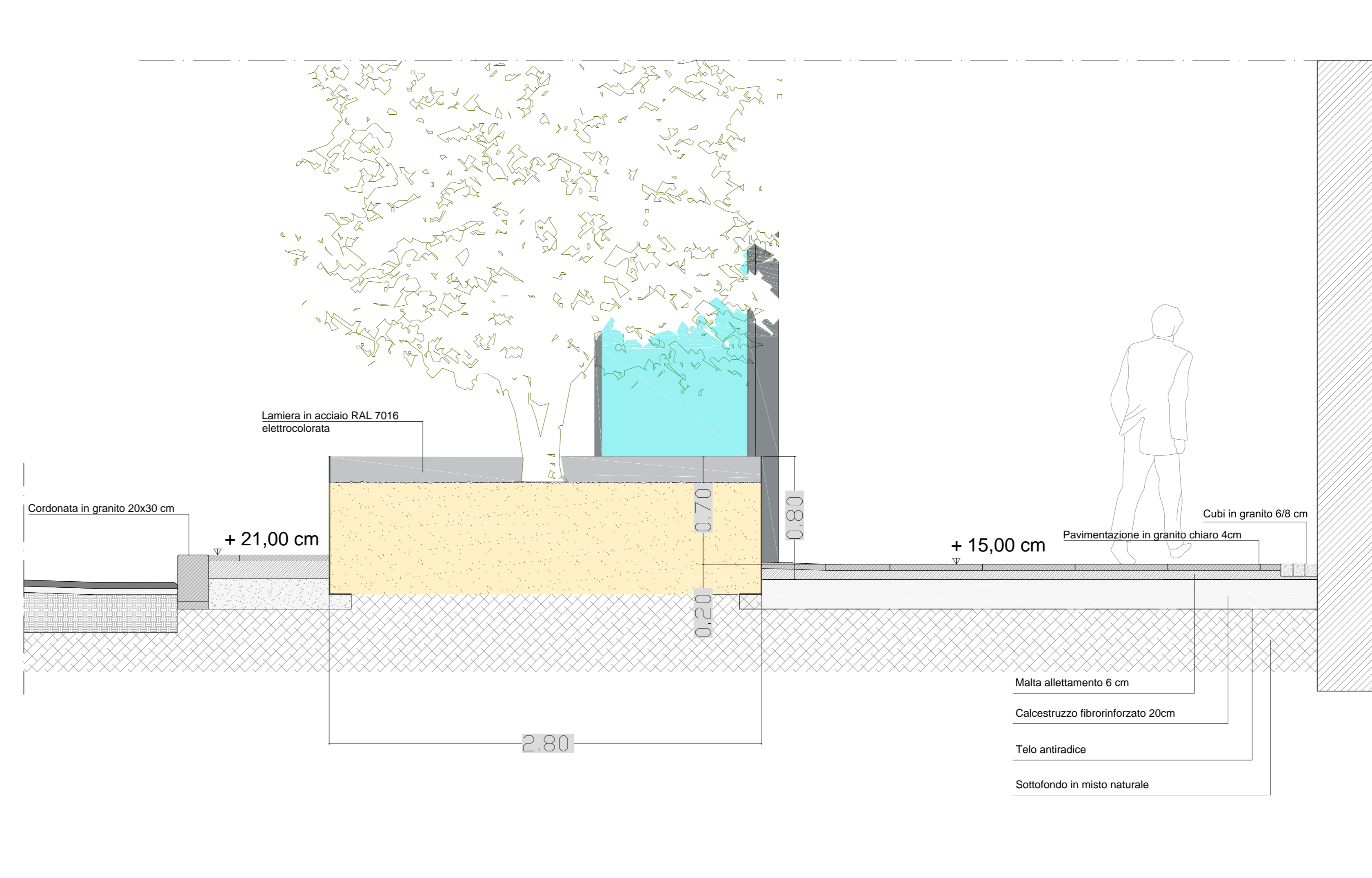
Sezione D-D'_scala 1:100
